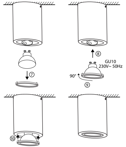
► DLO-AR-GU10-150
