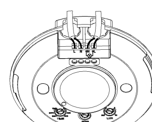
dráty ze strany
