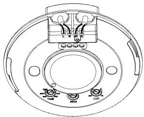
Górne wyprowadzenie przewodów zasilających
