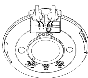
Boczne wyprowadzenie przewodów zasilających
