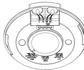
соединительные кабели снизу
