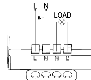
L - vodič pod proudem; N - neutrální napájecí kabel a neutrální zatížení (např. svítidlo); L "- zatížení drát (např. svítidlo)
