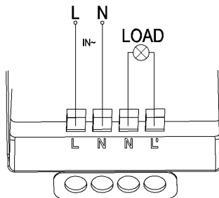
L – faza zasilająca N- przewód neutralny zasilania przewód neutralny obciążenia (np. oprawy) L' – przewód fazowy obciążenia (np. oprawy)
