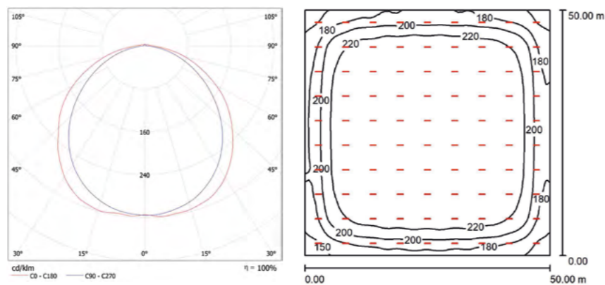
Pawilon handlowy; planowane natężenie 200lx; HLC2-120B-50B-840B
